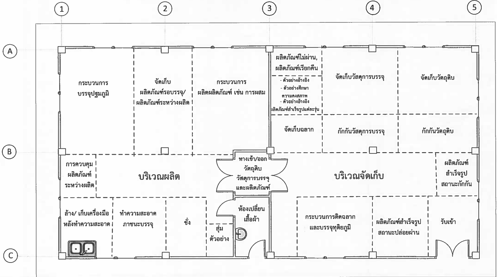
ตัวอย่าง แนวทางการจัดแบบแปลนสถานที่ผลิตผลิตภัณฑ์สมุนไพรที่มีกระบวนการผลิตความเสี่ยงต่ำและเป็นผลิตภัณฑ์สำหรับใช้ภายนอก
